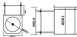
320 con pasillo técnico
