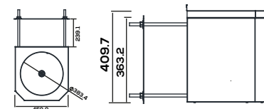
420 con pasillo técnico
